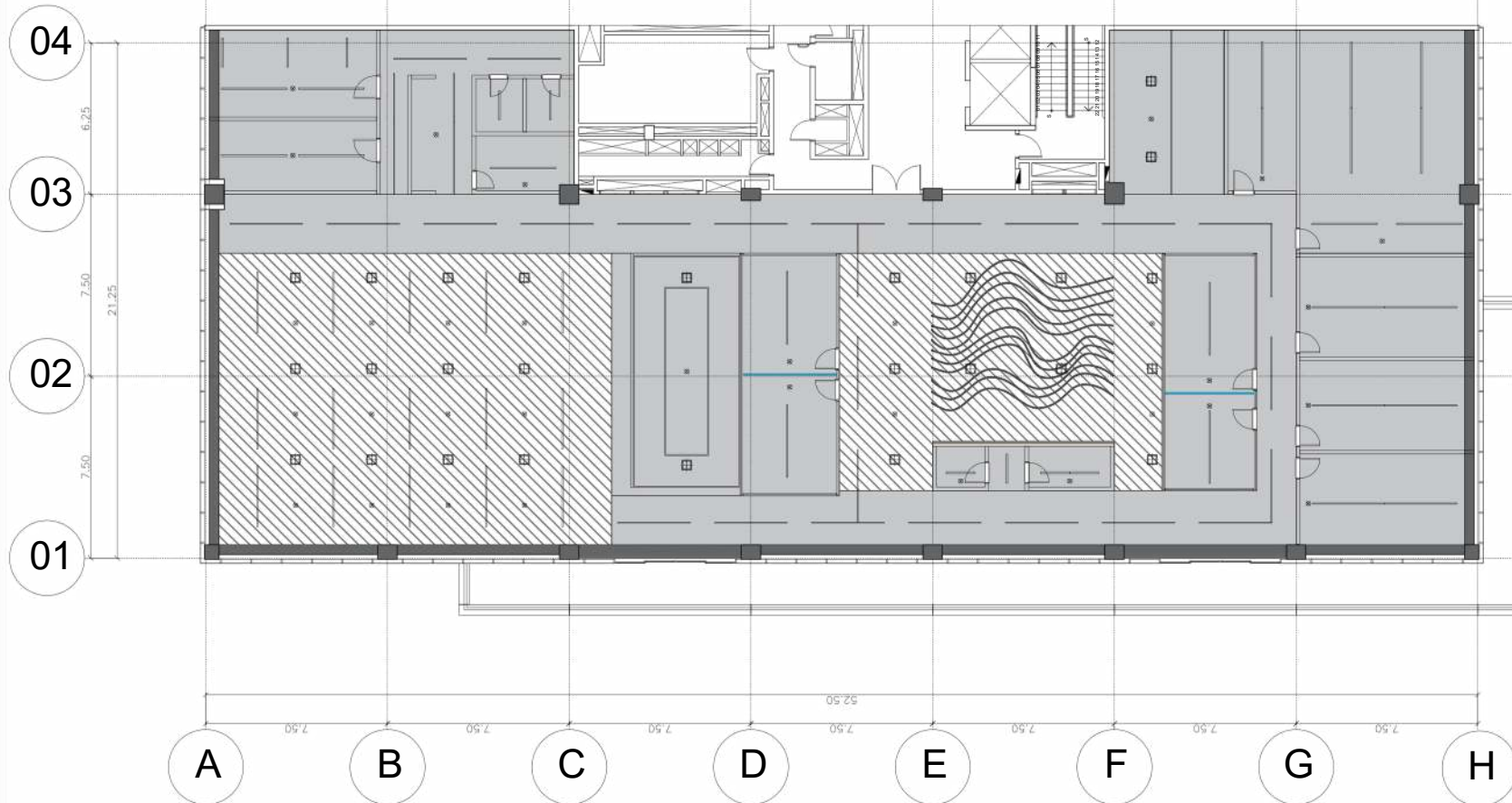
PLANTA DE FORRO ESC.: 1:200
